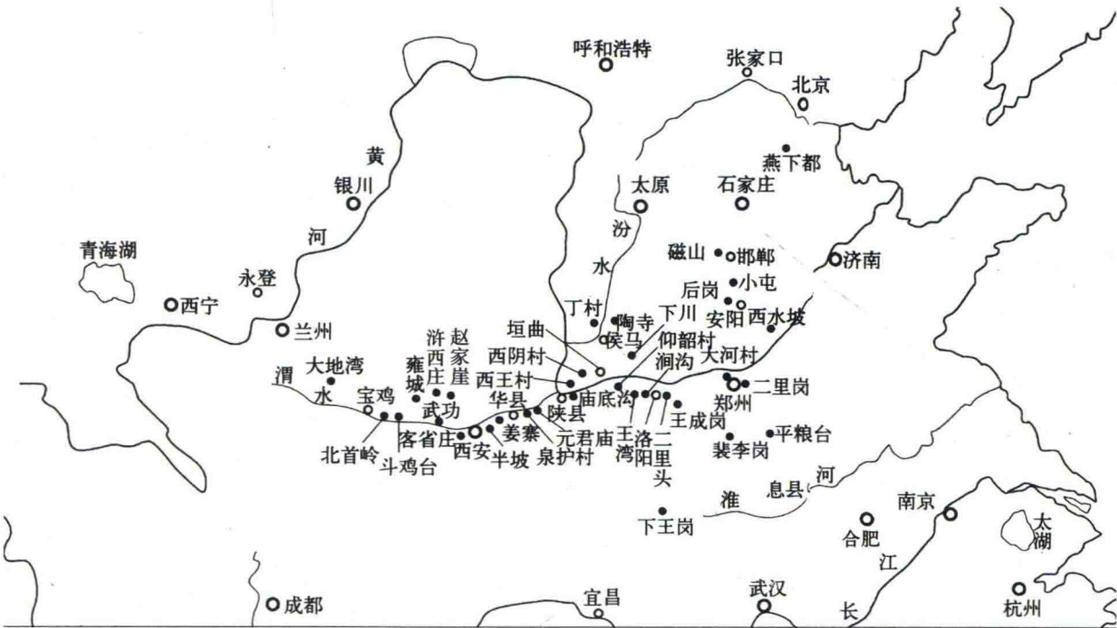
文化区系中的中原区系示意图《中国文明起源新探》
