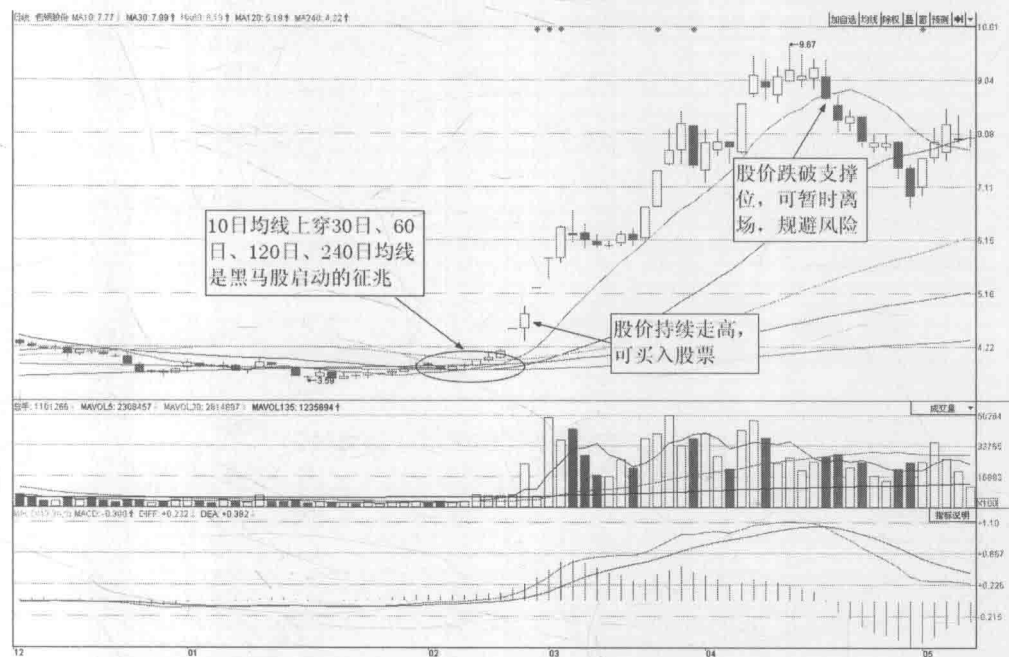
图 1-1 包钢股份 (600010) 日 K 线图
