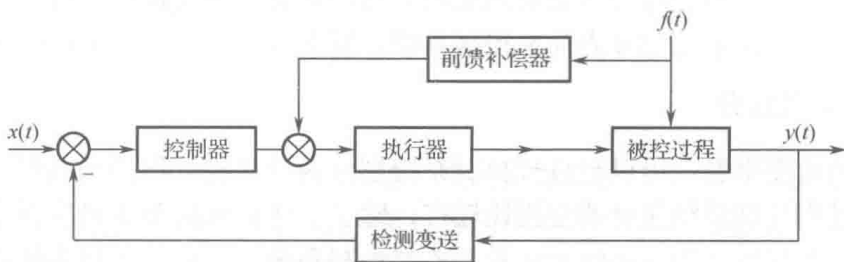
图 1-5 前馈-反馈复合控制系统方框图
