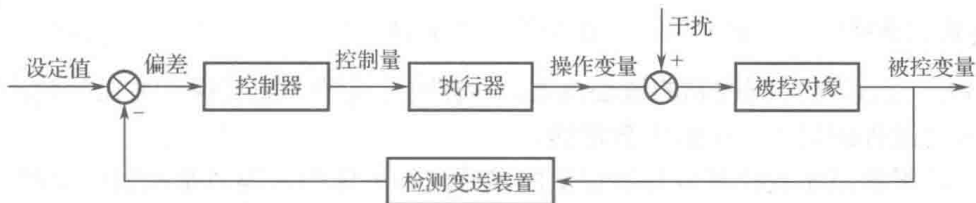
图 1-3 反馈控制系统方框图
