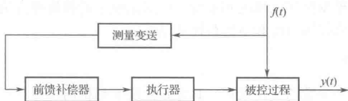
图 1-4 前馈控制系统方框图
