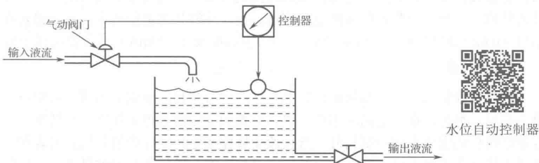
图 1-1 储液罐液位控制系统
