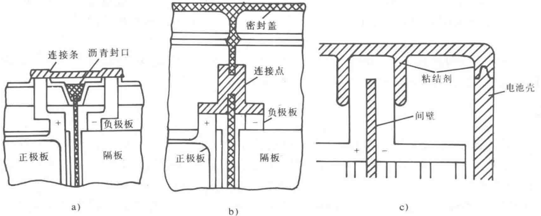
图 1-2 单体电池的连接方式
