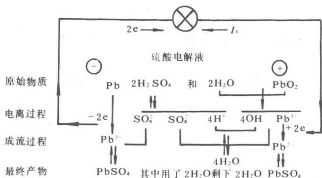
图 1-3 蓄电池的放电过程
