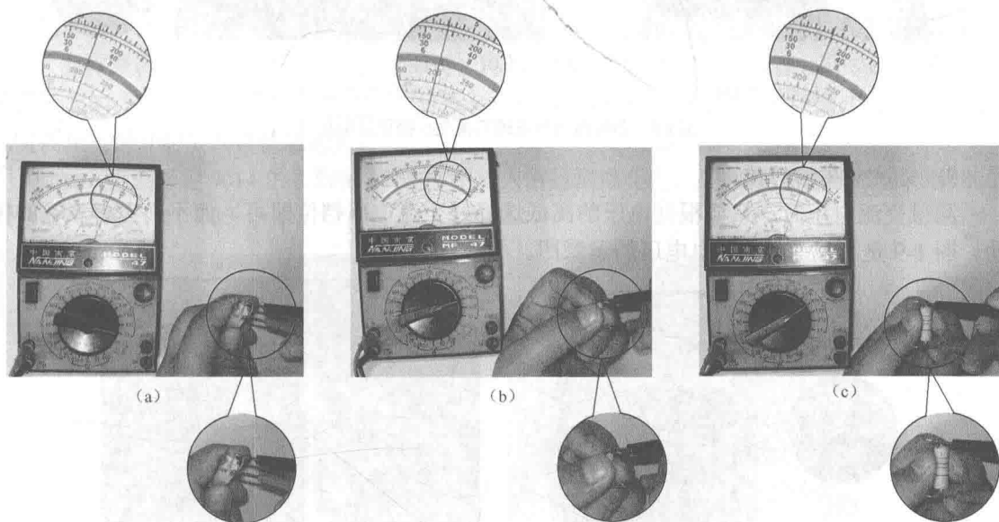
图 1-7 指针型万用表的电阻挡使用示意图
