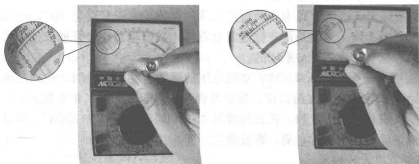
图 1-4 指针型万用表表针复位的调整
