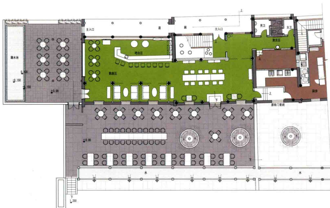
一层平面布置图
