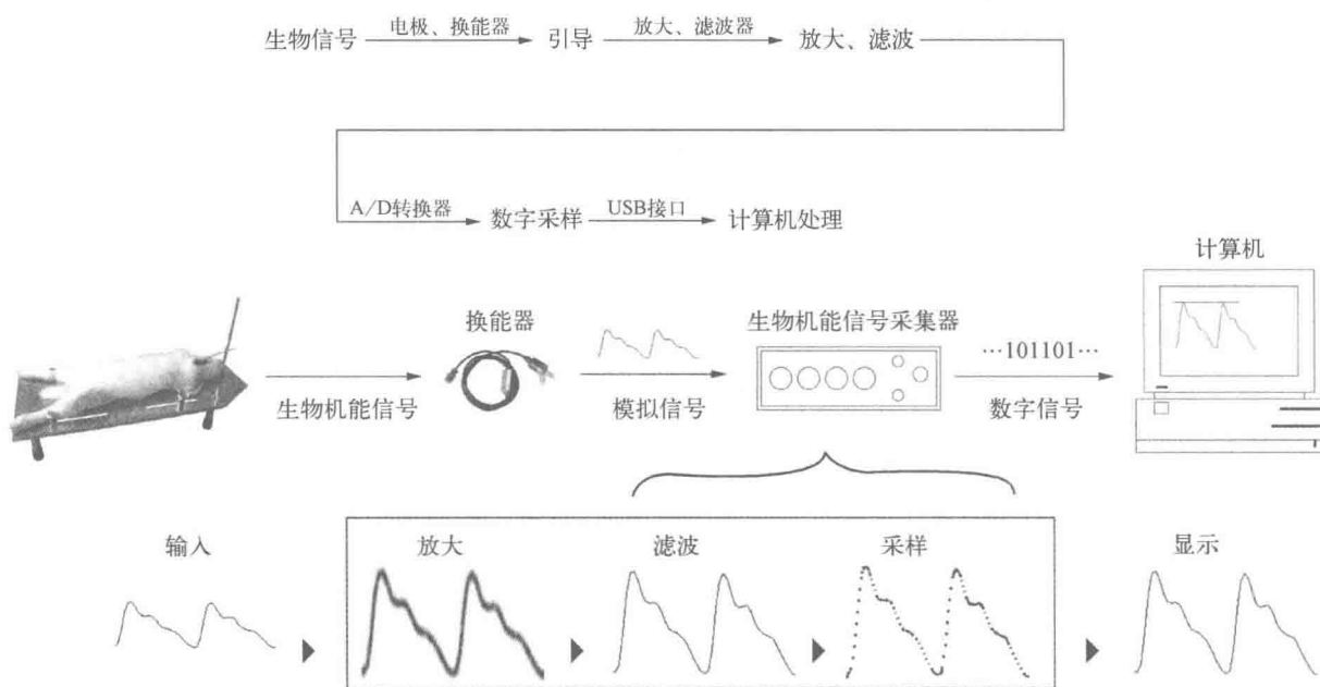
图 1-1 生物信号采集与处理系统原理
