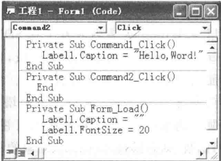
图 1.3 例 1.1 的程序代码
