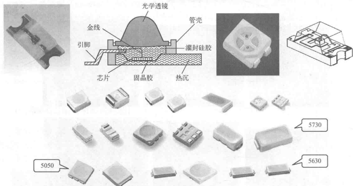
图 1-7 SMD 封装的外形与结构
