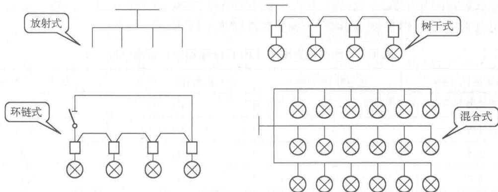
图1-4 接线方式
