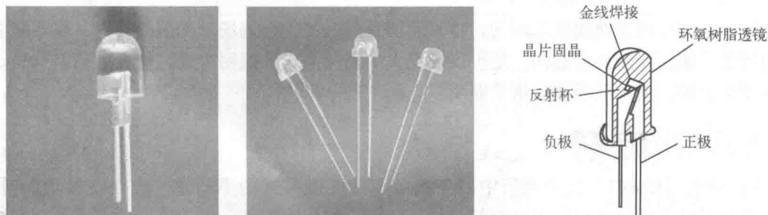
图 1-5 插件型封装的外形与结构
