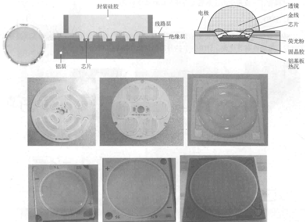
图 1-6 COB 封装的外形与结构
