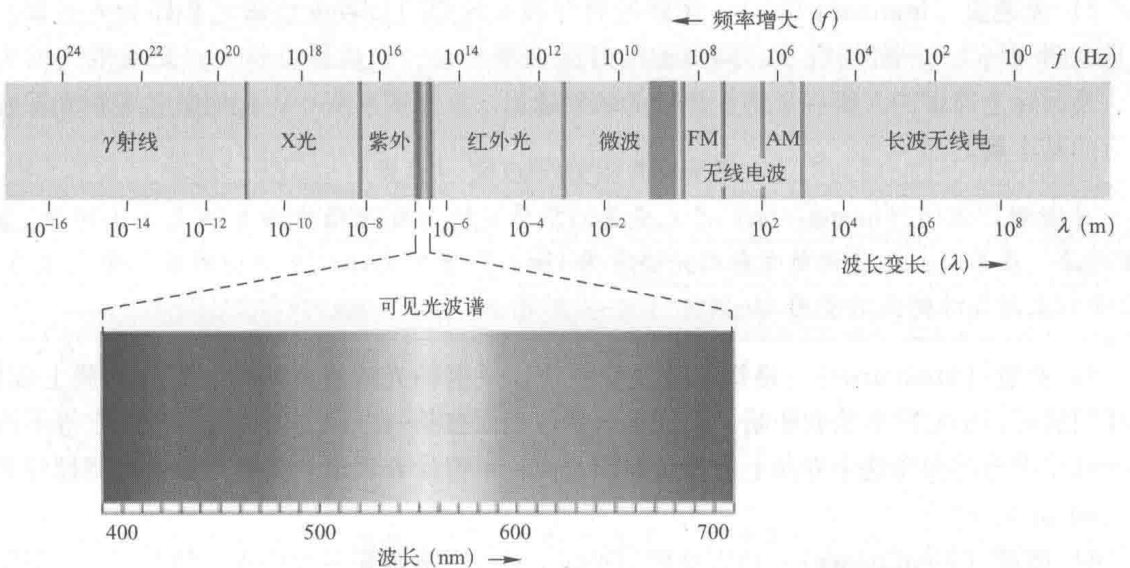
图 1-2 电磁波的辐射波谱
