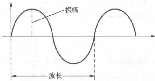
图 1-1 波长、振幅及频率之间的关系
