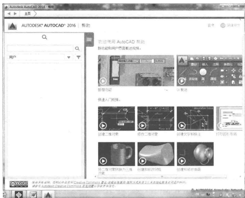
图 2-9 帮助窗口
