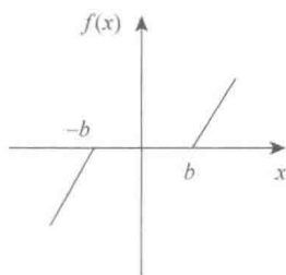
图 1.4 齿侧间隙与力的关系图
