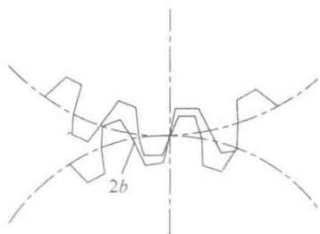
图 1.3 齿侧间隙
