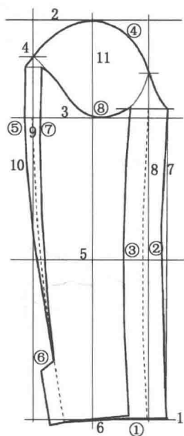
图 1-2 衣袖基础线与结构线
