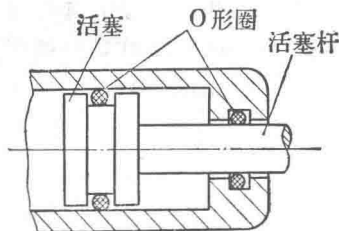
图 1-1 O形圈及其安装沟槽
