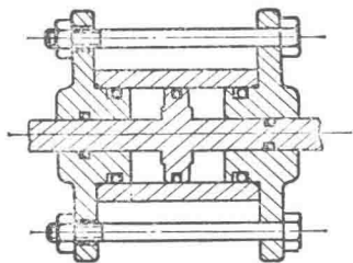
图 1-3 用于空气压缩机中的 O 形圈
