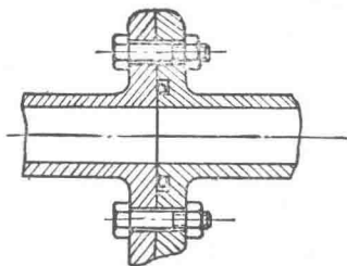
图 1-4 用于真空装置法兰盘 处的 O 形圈
