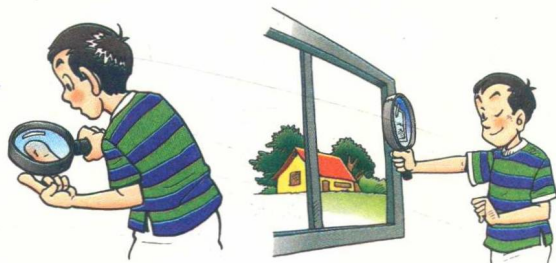
图3 透过放大镜看，物体总是放大的吗？
