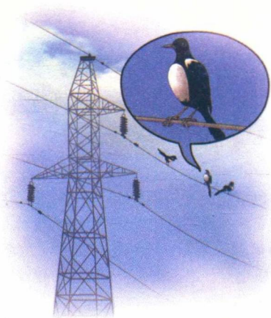
图8 架空的高压输电线是裸露的，为什么小鸟却能若无其事地停在电线上呢？
