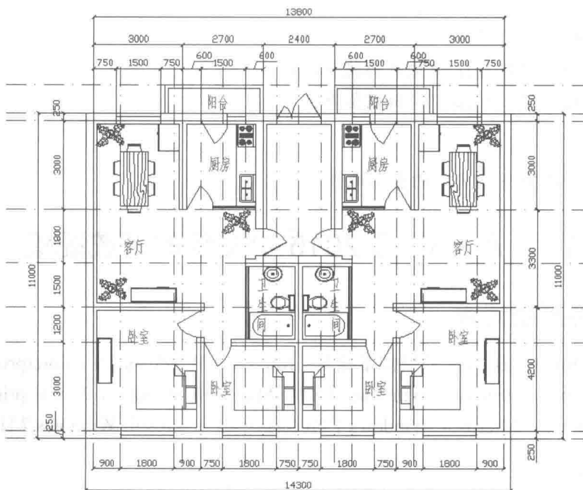
图 1-1 平面图
