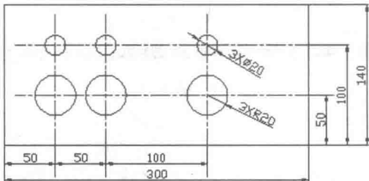
图 1-3 标注尺寸图
