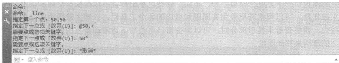
图 1-10 “命令行”窗口
