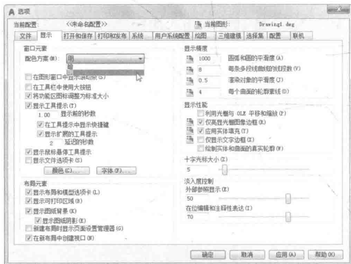
图 1-3 “选项”对话框
