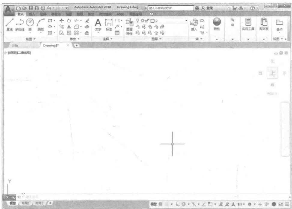
图 1-4 “明”界面
