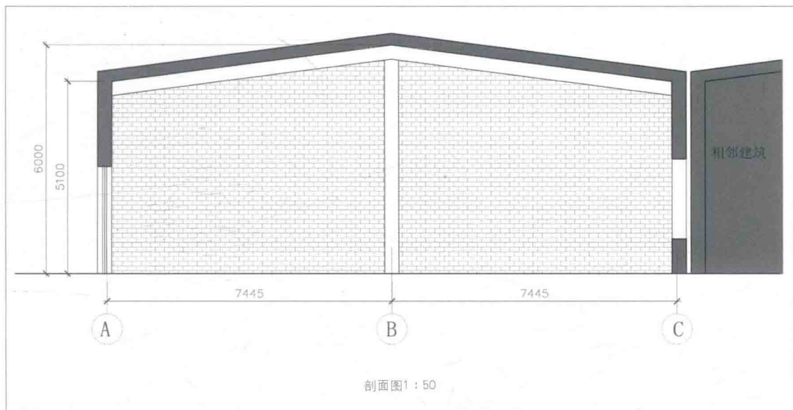
图2-2 原始剖面图
