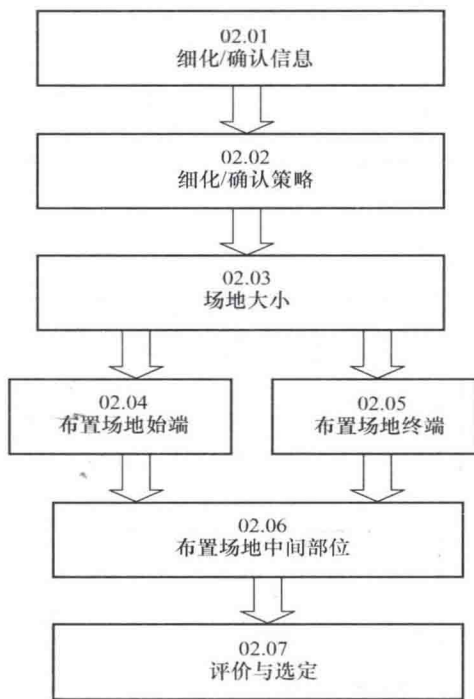
图 1-4 前空间规划（FacPlan 的第二层次作业）
