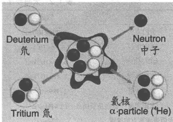
图 1.1 太阳核聚变反应
