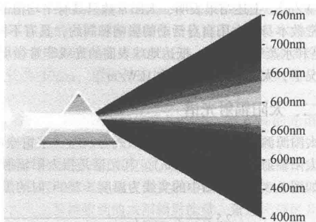
图 1.2 太阳可见光谱
