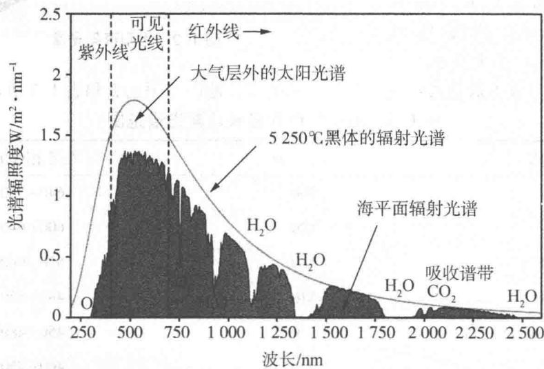
图 1.3 太阳辐射光谱
