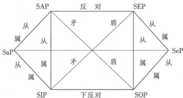
图 1—3 六角阵图
