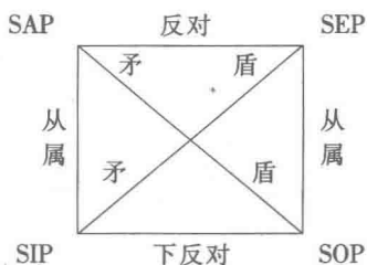
图 1—2 逻辑方阵图
