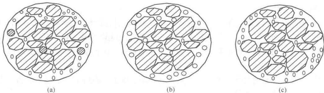
图 1K411014 沥青混合料的结构组成示意图
