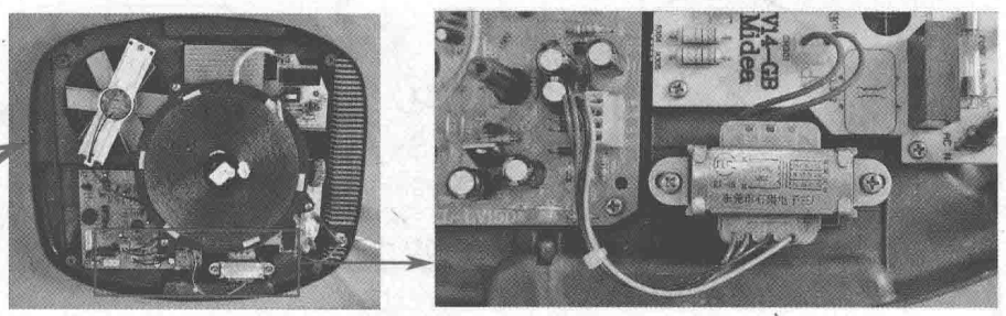
为了满足电子元件工作要求，通过交/直流变换电路实现市电交流到直流的变换
