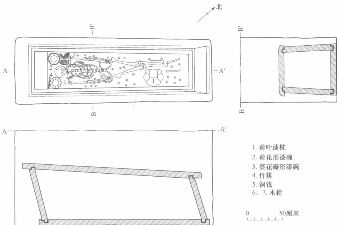
图三 M2 平、剖面图
