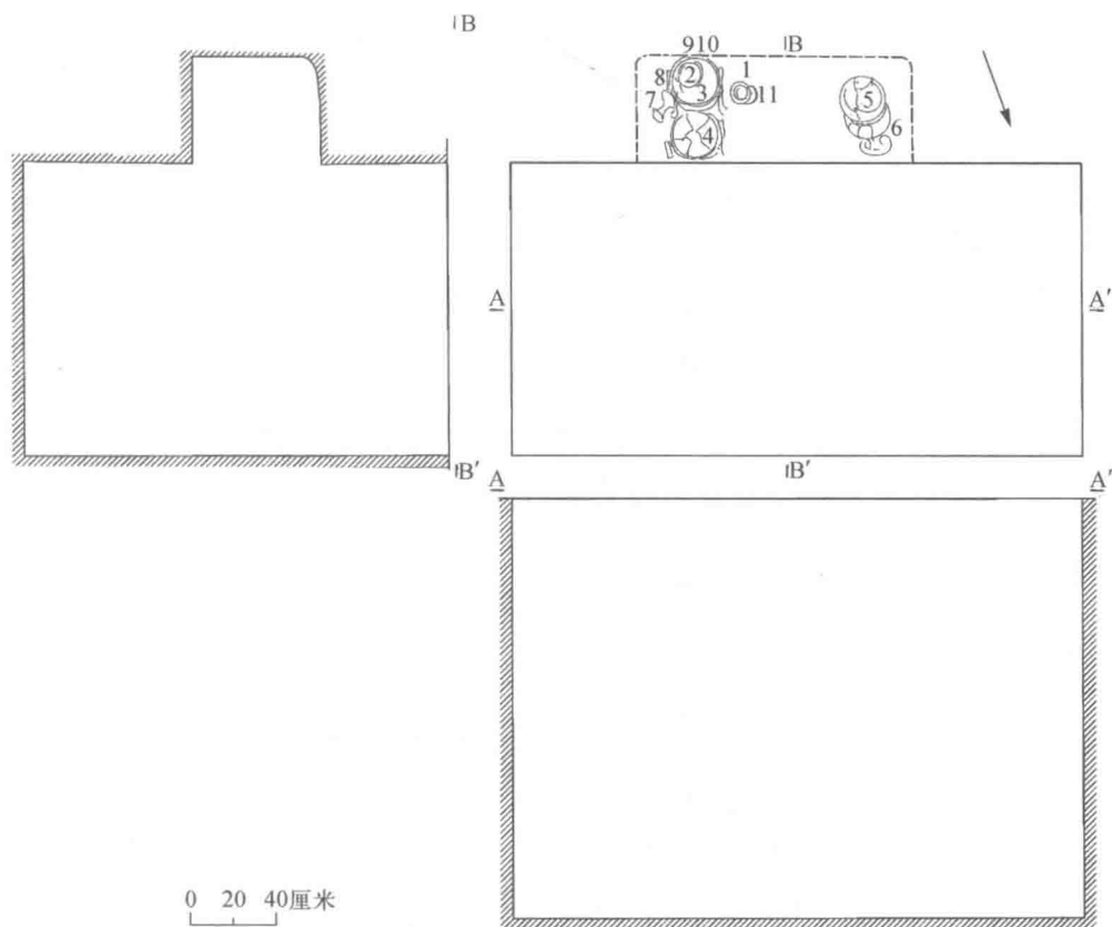
图 730-1 M753 平、剖面图
