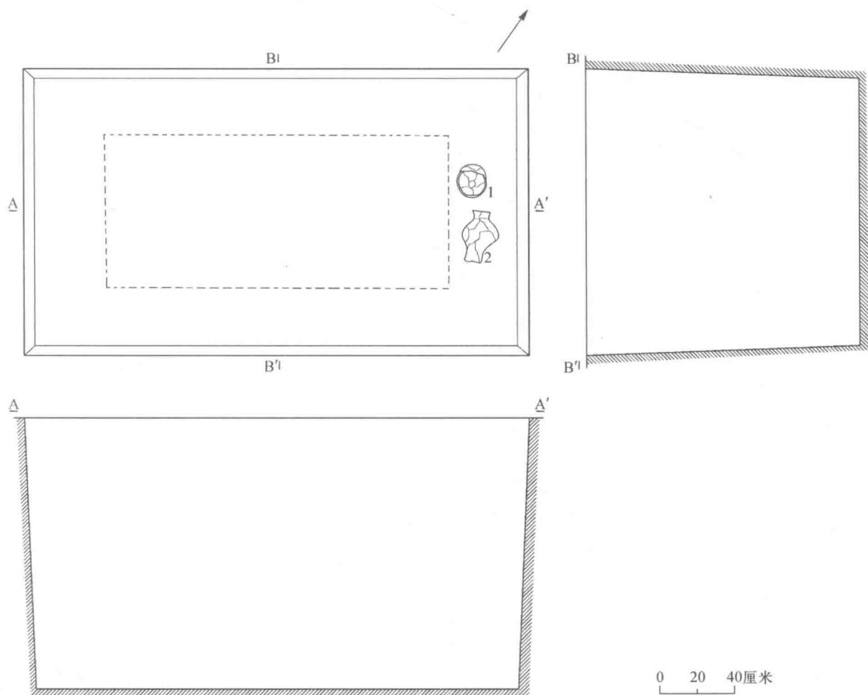
图 734-1 M758 平、剖面图
