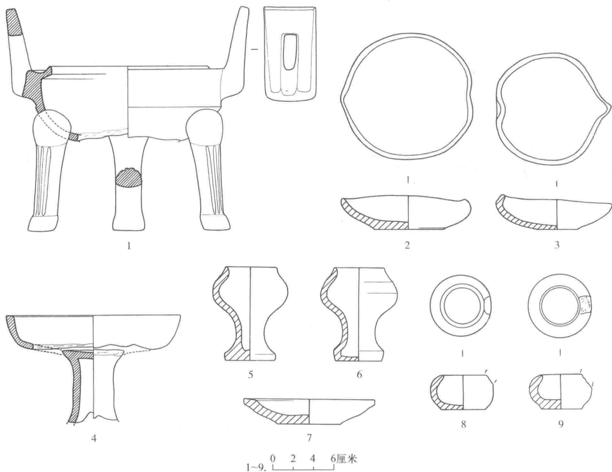
图 730-2 M753出土器物
