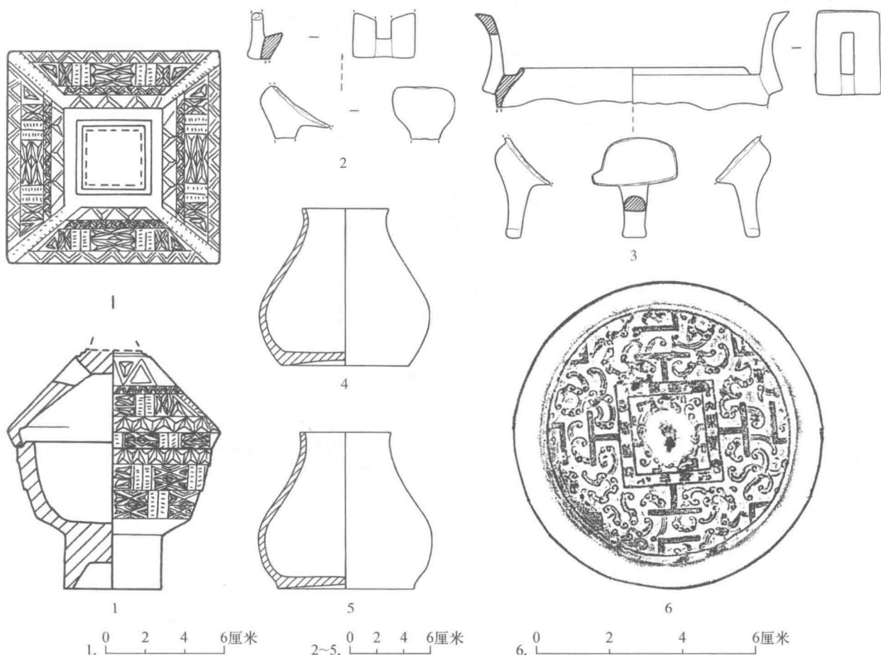
图732-2 M755出土器物(一)
