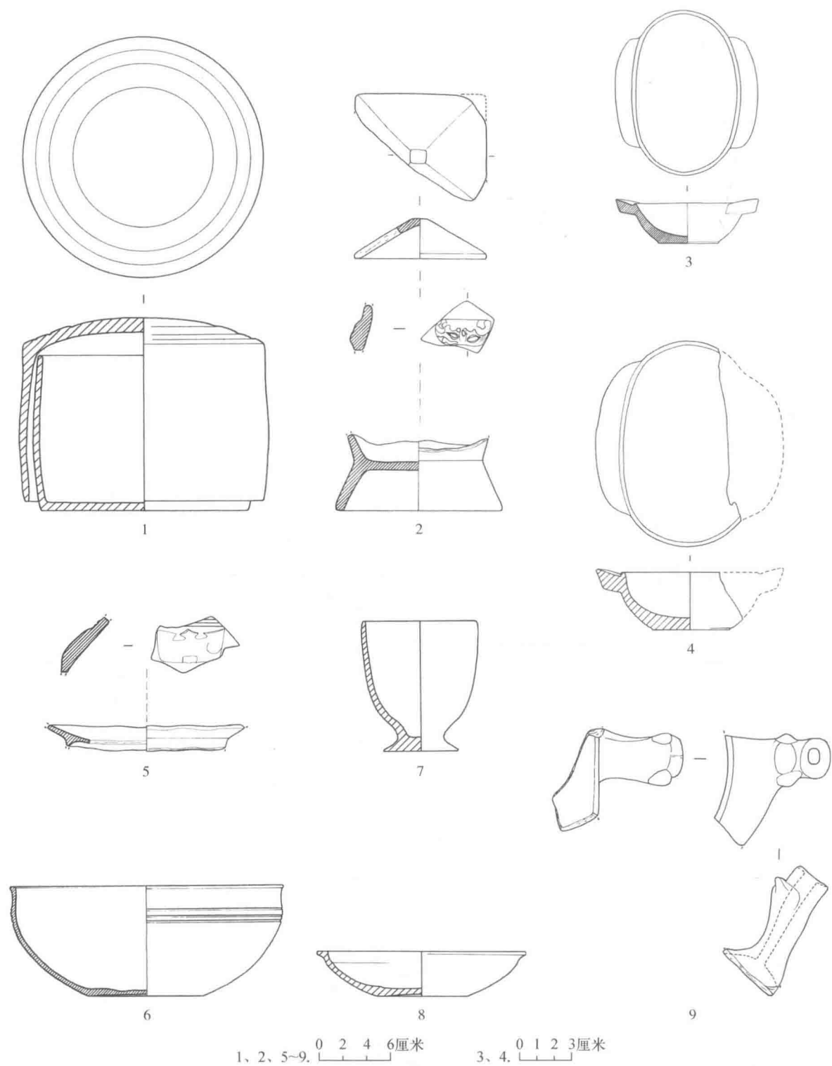
图 732-3 M755 出土器物 (二)
