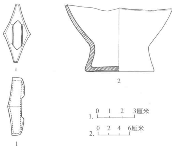
图 729-2 M752出土器物
