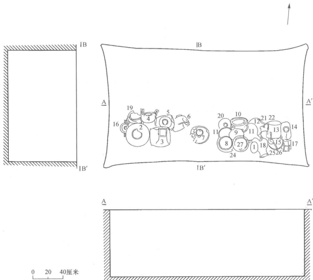
图733-1 M756平、剖面图
