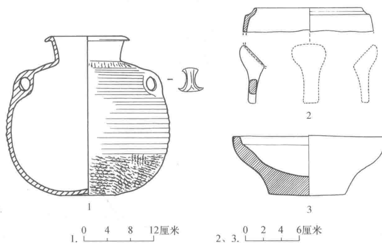
图 731-2 M754 出土器物
