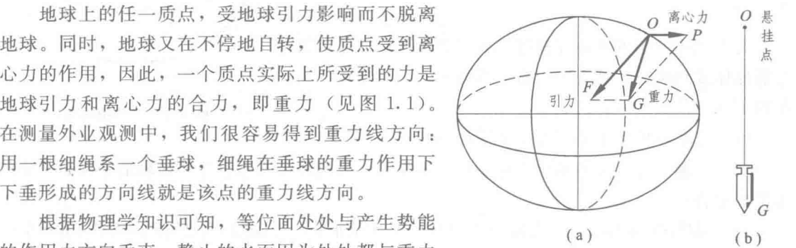
图 1.1 重力与重力线
