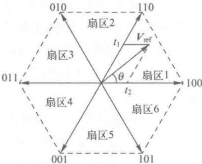
图 1-12 三相电压型电力电子变换器空间矢量 PWM
