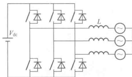
图 1-6 三相电压型逆变器拓扑结构
