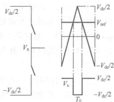
图 1-10 电压型电力电子变换器桥臂通过 PWM 实现参考电压逼近的方法
