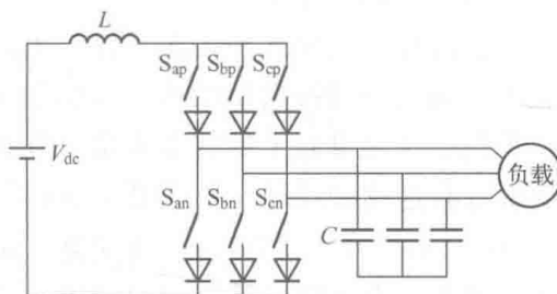
图 1-7 三相电流型逆变器结构
