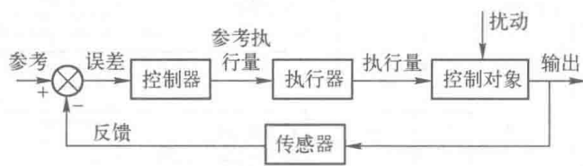
图 1-8 一个典型的控制系统框图
