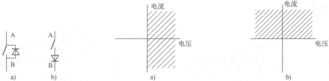
图 1-1 电力电子变换器中的两种典型开关 a) 电流双向开关 b) 电压双向开关
