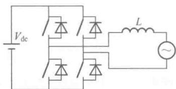
图 1-5 单相电压型逆变器拓扑结构
