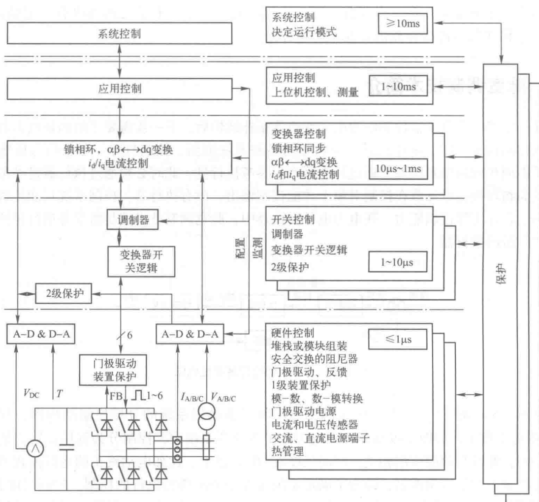
图 1-9 电力电子系统的分层控制图 [6,7]
