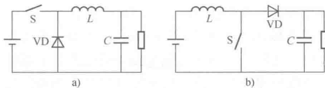
图 1-4 两种典型的直流-直流变换器拓扑
