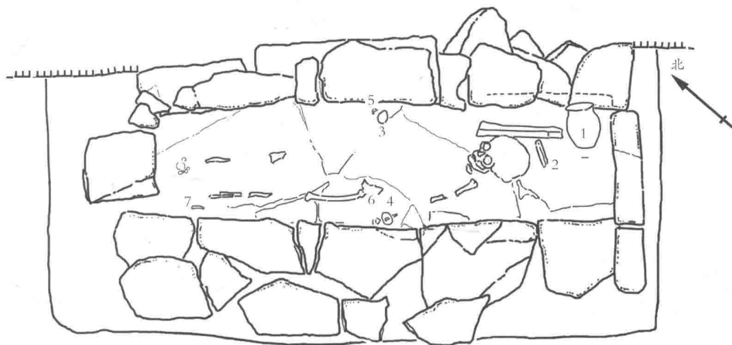
图九 M1 平面图
