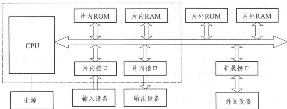
图 1-2 单片机系统结构框图
