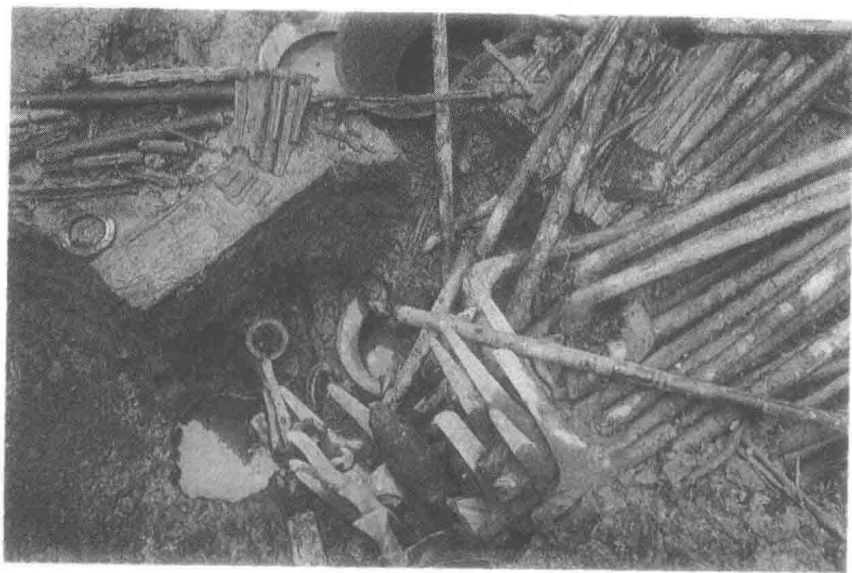
图九 M113 腰坑局部
