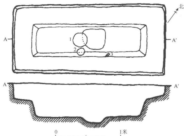
图一二 M52 平、剖面图
