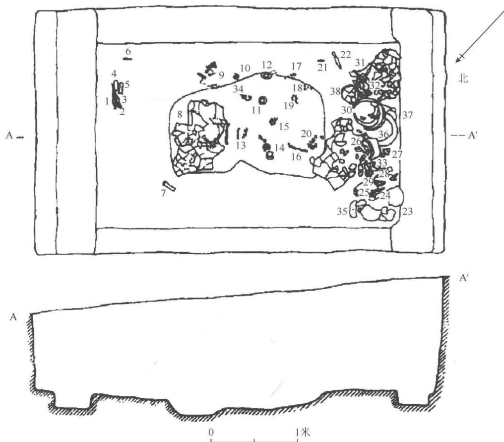
图一〇 M30 平、剖面图
