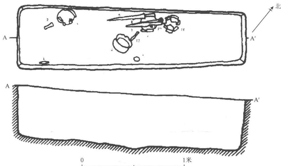
图一一 M194 平、剖面图
