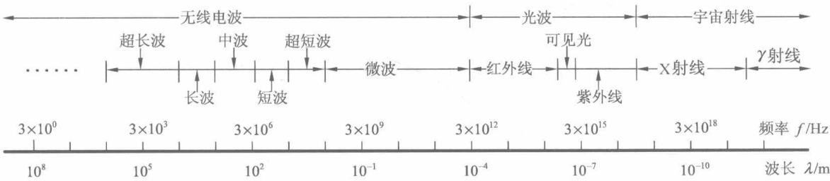
图 0-1 微波频段在电磁波频谱中的位置
