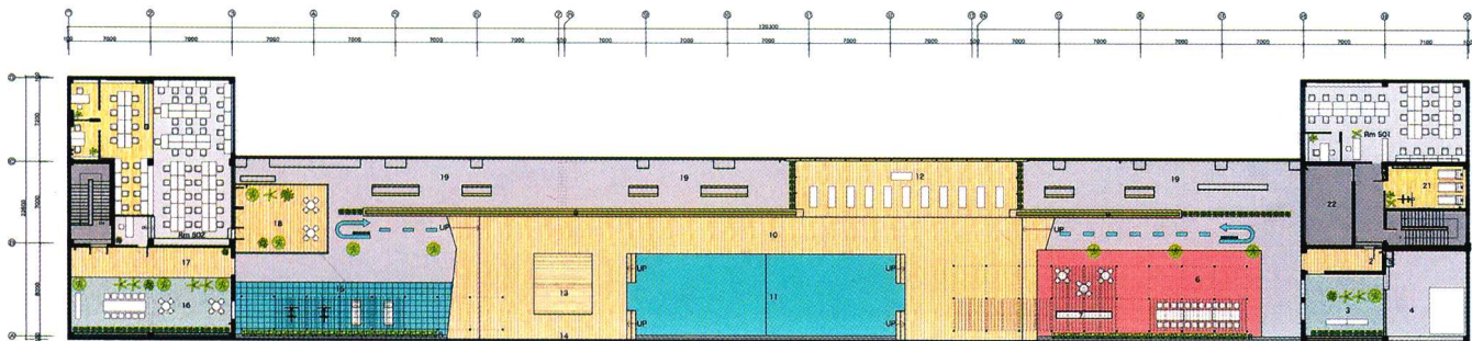
屋顶层平面图 Roof Floor Plan
