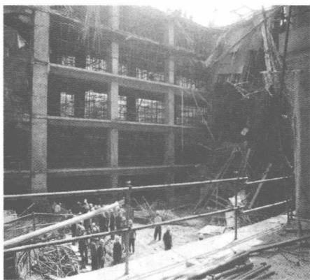
图 1.1-7 北京模架垮塌事故
