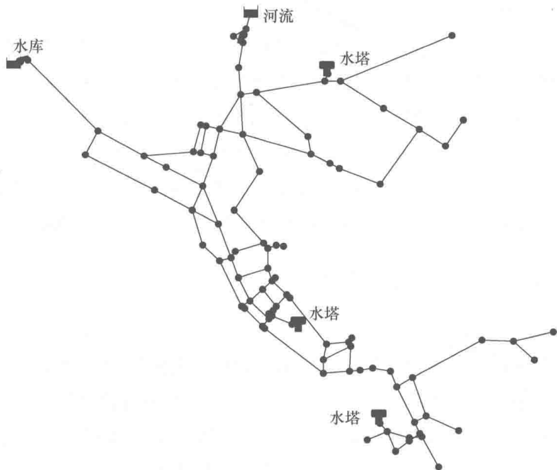
图 1-2 管网输配系统的组成
