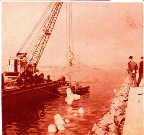
▷ 投锥筑堤
