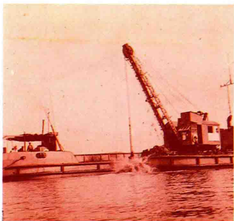
▷ 冷库施工
