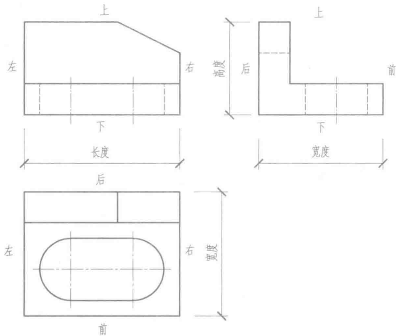
图 1-13 三面投影图
