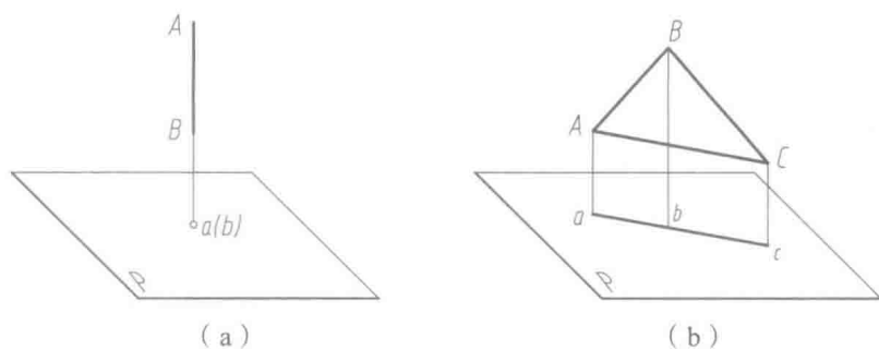
图 1-6 积聚性
