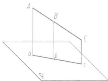
图 1-8 从属性、等比性
