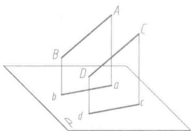
图 1-7 平行性、等比性
