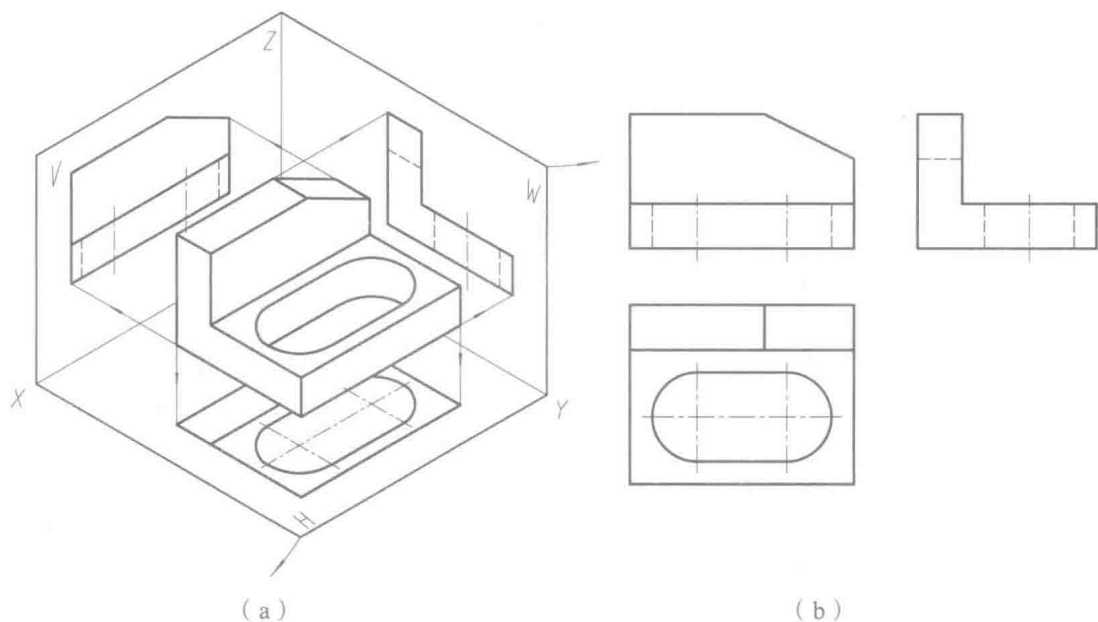
图 1-12 物体的三视图
