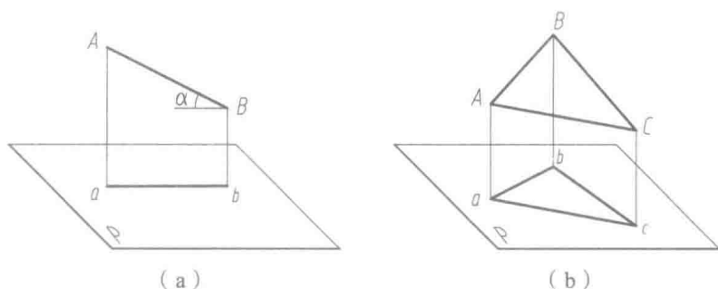
图 1-5 类似性
