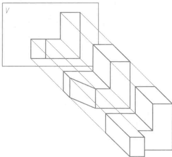
图 1-9 一个投影不能确定物体形状
