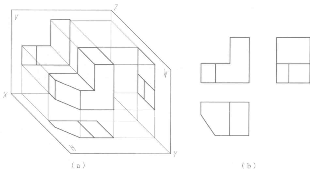
图 1-10 多面投影图
