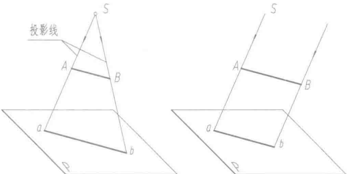
图 1-2 两种投影法
