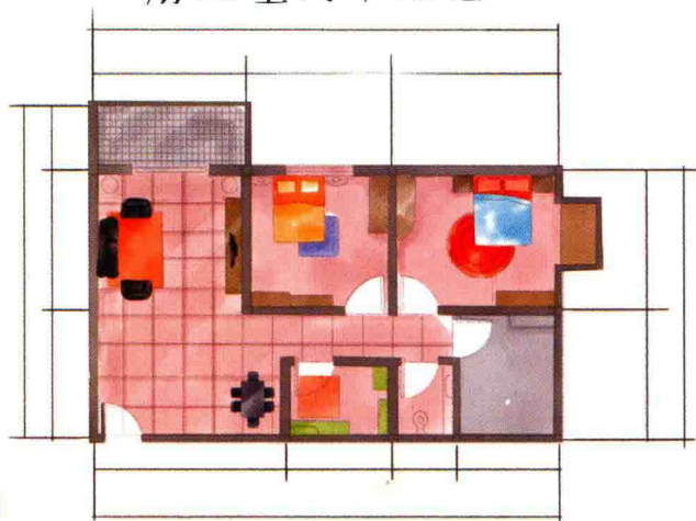
房屋室内平面图
