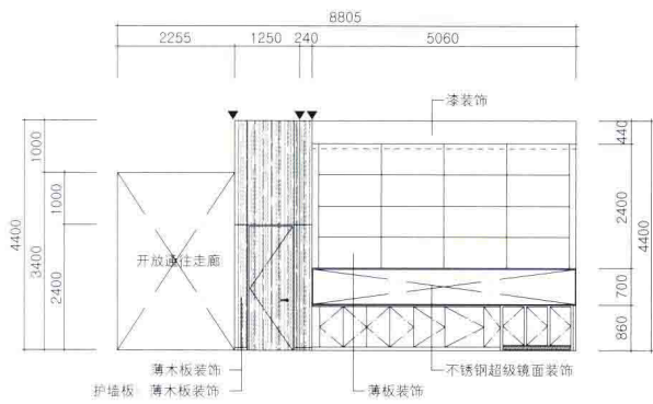
立面图G
