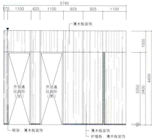
立面图K
