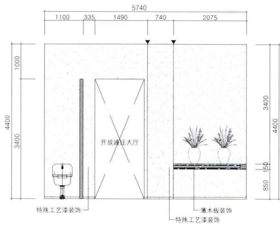
立面图J
