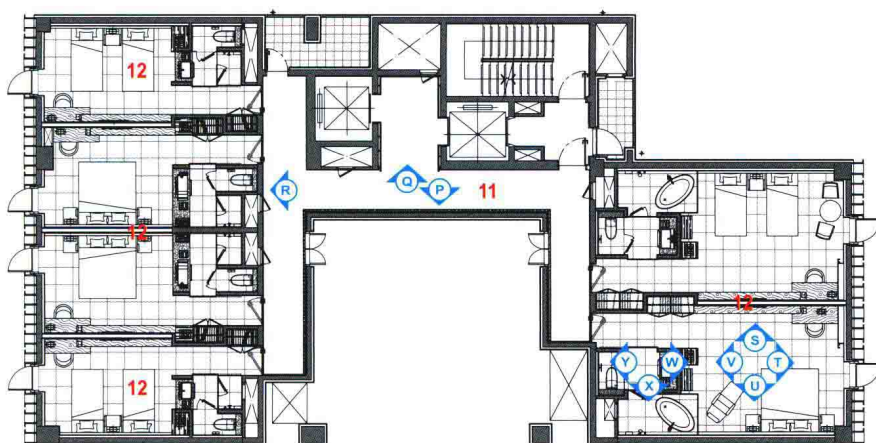
二至八层平面图
