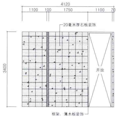
立面图N
