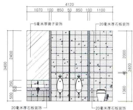
立面图O
