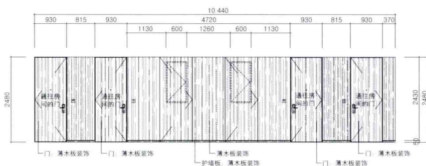
立面图R
