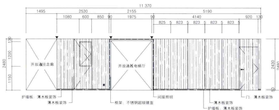
立面图Q
