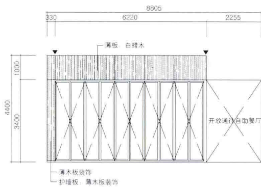
立面图H
