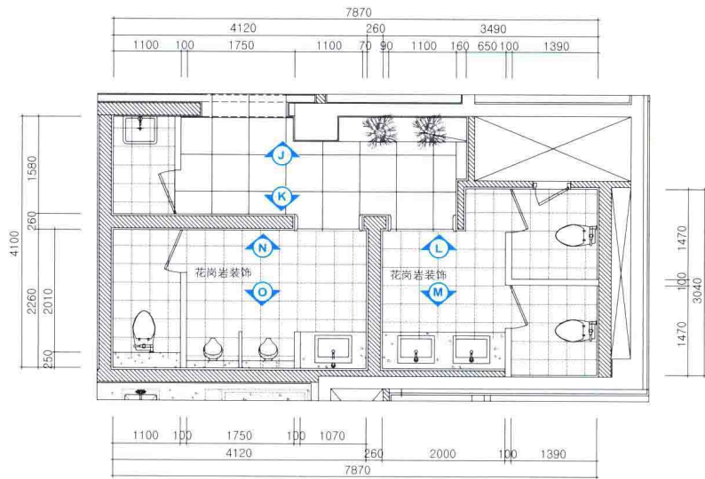
厕所平面图
