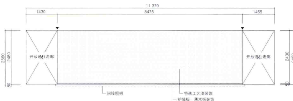
立面图P
