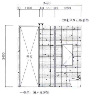
立面图L
