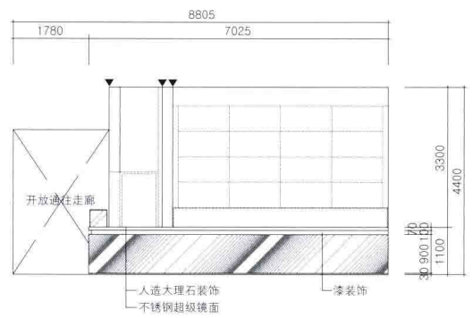
立面图G'
