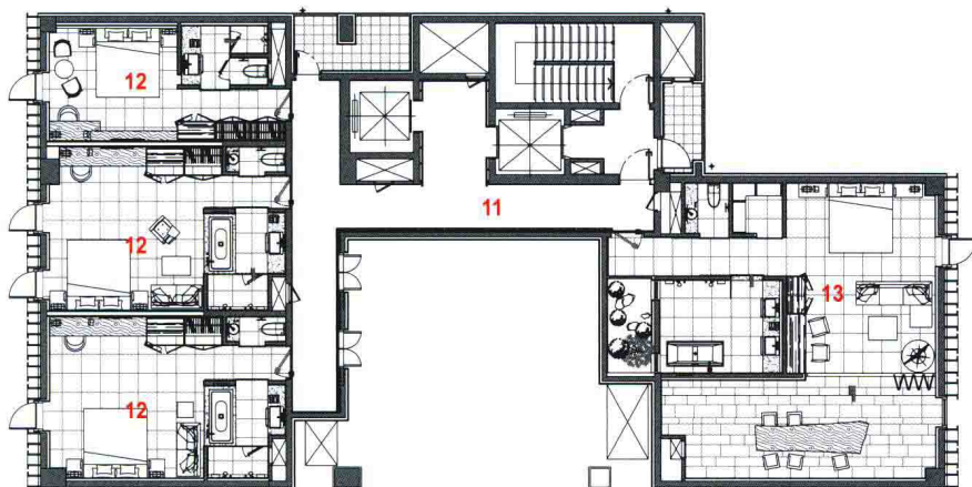
九层平面图
