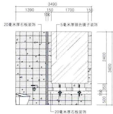
立面图M
