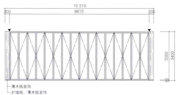
立面图I
