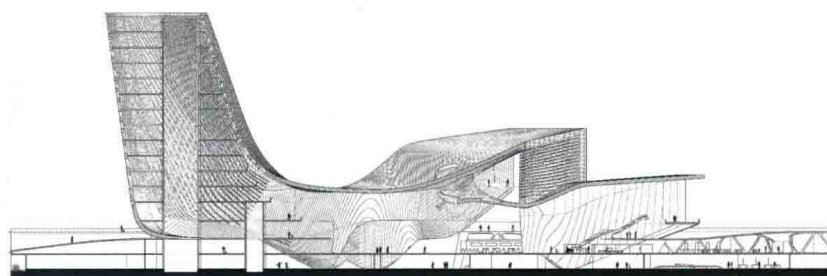
LONGITUDINAL SECTION 剖面
