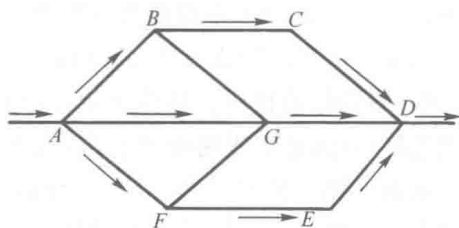
图 1-3 环状管网
