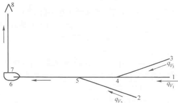
图 1-1 枝状管网
