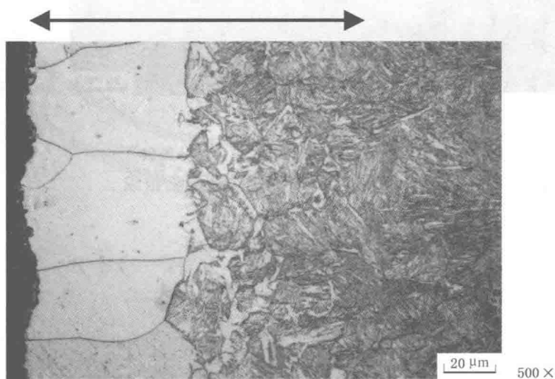
处理工艺: 先 870 °C 加热 20 min 油淬, 之后 440 加热 90 min 空冷; 组织说明: 白色铁素体部分为完全脱碳区, 含有片状铁素体区为部分脱碳
