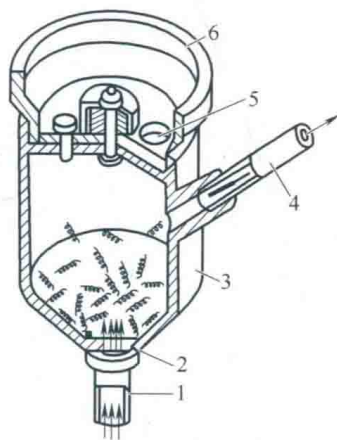
图 1-9 小型散料的标准供料设备——振动盘
