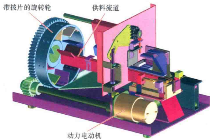
图 1-11 旋转式螺钉供应机
