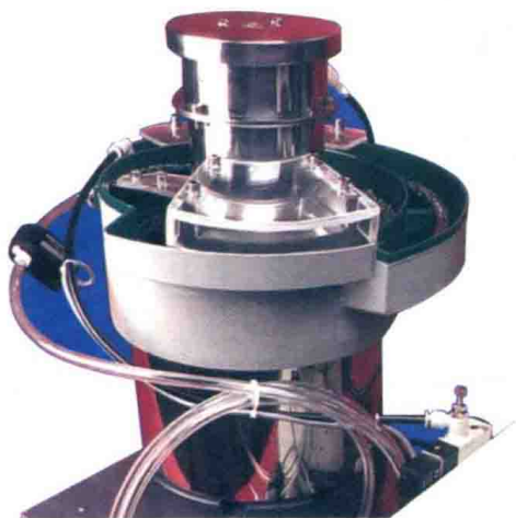
图 1-13 弹簧供料机
