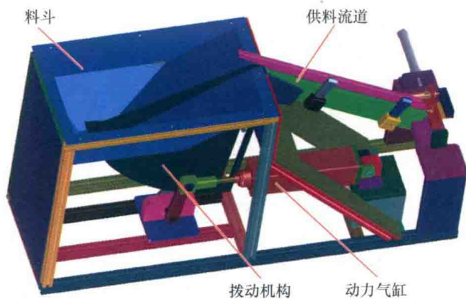
图 1-12 往复式螺钉供应机
