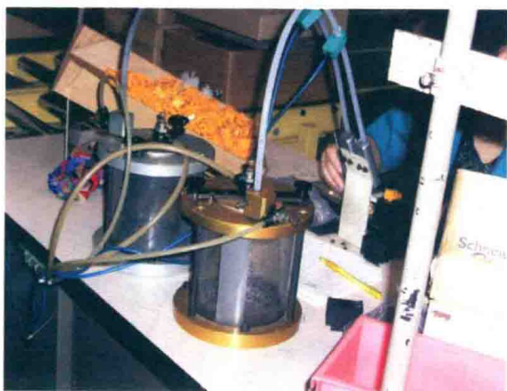
图 1-10 气吹式弹簧供料设备和原理
