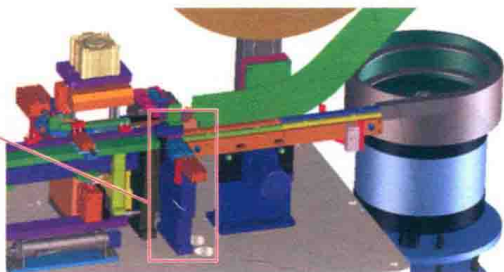
图 1-21 设备上的分离机构
