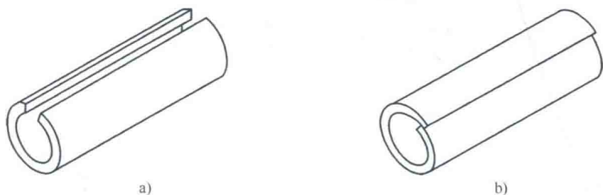
图1-5 滚子销产品结构
