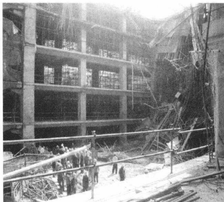
图 1.1-7 北京模架垮塌事故
