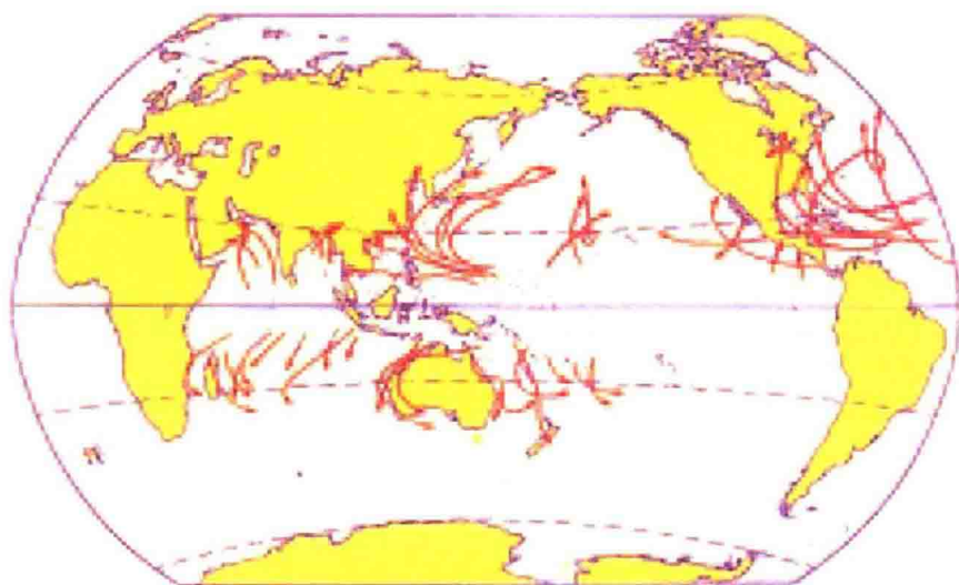
图 1-2 世界热带气旋主要路径示意图
