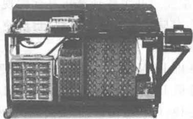
图 1-7 Atanasoff-Berry 计算机
