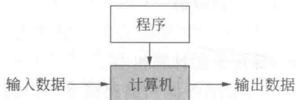
图 1-2 图灵模型
