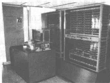
图 1-8 Z-3 型计算机
