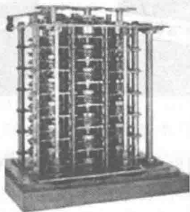
图 1-5 差分机
