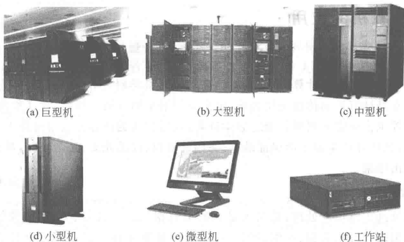
图 1-15 计算机分类
