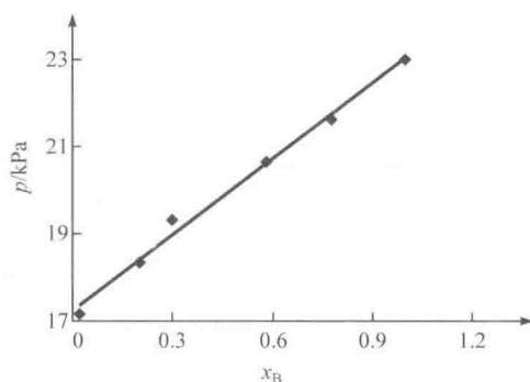
图 1.3 物质 B 的摩尔分数浓度与蒸气压的关系 (25°C)
