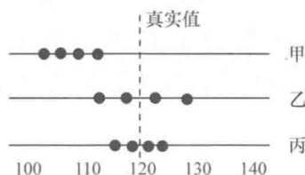
图 1.1 准确度与精密度的关系
