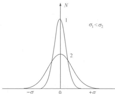
图 1.2 偶然误差正态分布曲线
