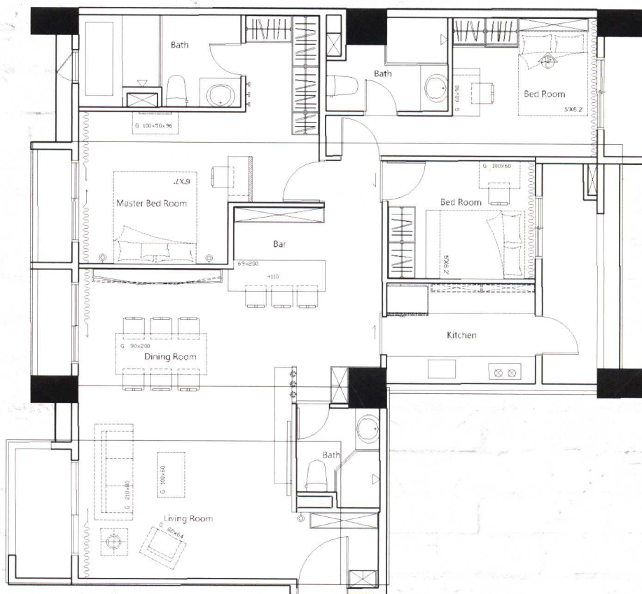
平面布置图
