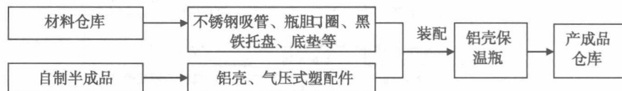
图 1-8 装配车间装配成铝壳气压保温瓶，铝壳气压式保温瓶生产工艺流程
