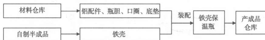
图 1-6 装配车间装配成铁壳保温瓶，铁壳保温瓶生产工艺流程
