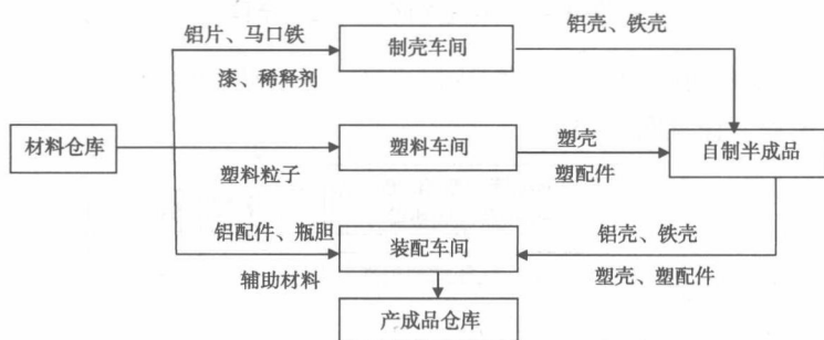
图 1-3 塑料车间生产工艺流程
