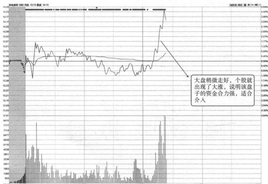
分时图
