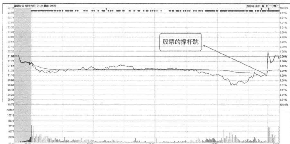
分时图
