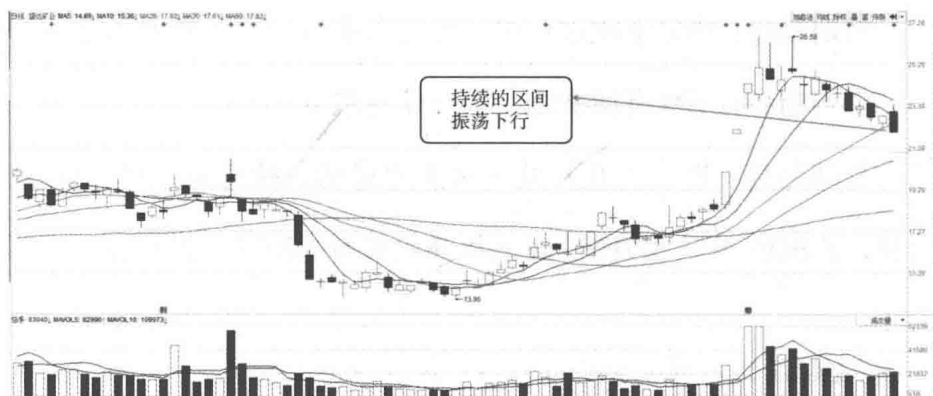
日K线图
