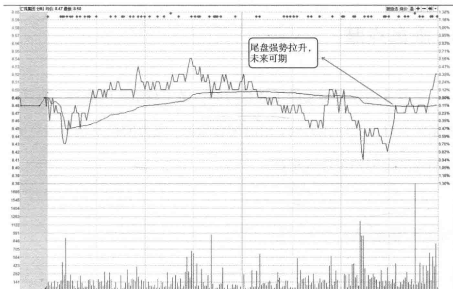
分时图
