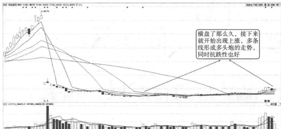
日K线图
