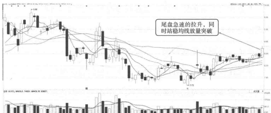
日K线图
