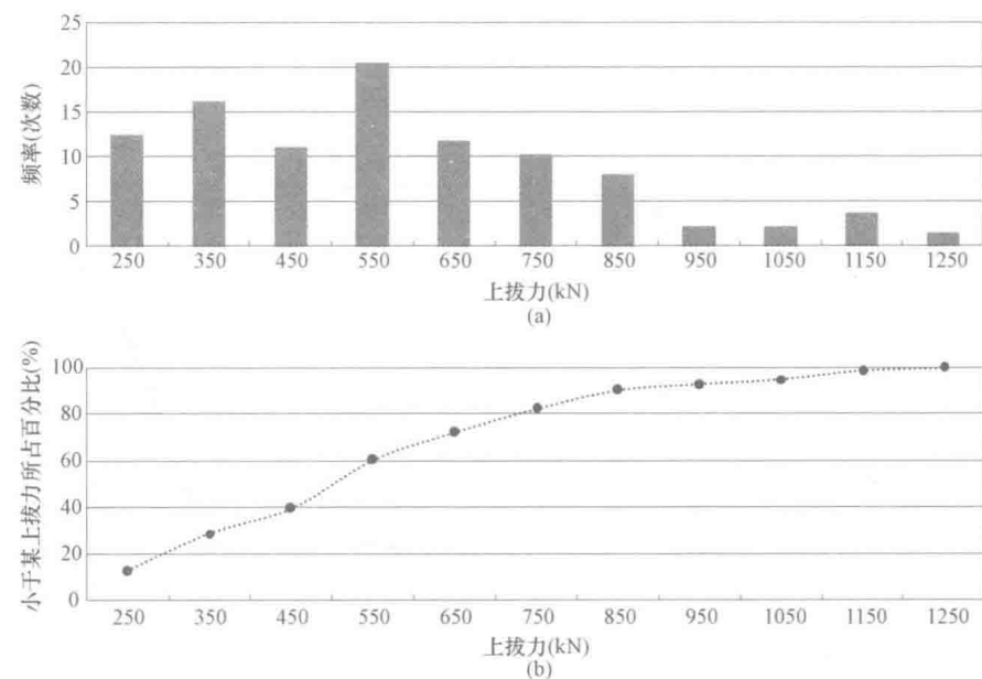
图 4.2-4 330kV 电压等级直线塔基础上拔力分布直方图及累积分布曲线 (a) 基础上拔力分布直方图; (b) 基础上拔力累积分布曲线
