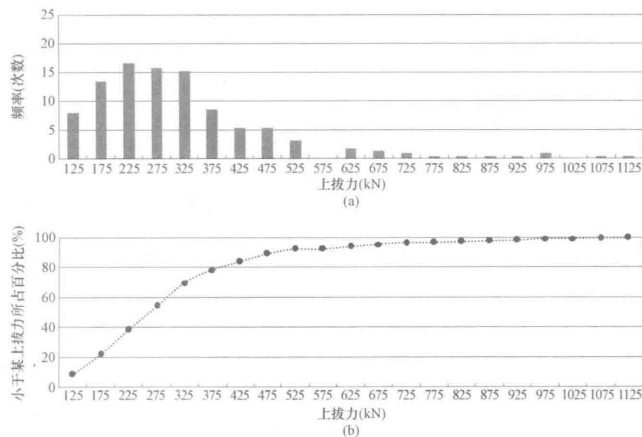
图 4.2-2 110kV 电压等级直线塔基础上拔力分布直方图及累积分布曲线 (a) 基础上拔力分布直方图; (b) 基础上拔力累积分布曲线
