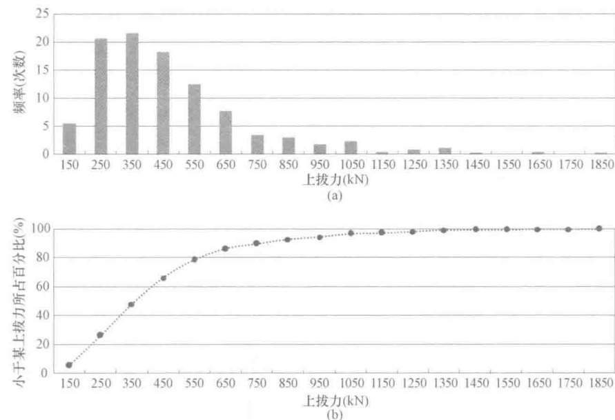
图 4.2-3 220kV 电压等级直线塔基础上拔力分布直方图及累积分布曲线 (a) 基础上拔力分布直方图; (b) 基础上拔力累积分布曲线
