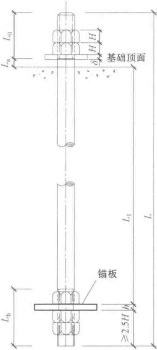
图 4.4-1 地脚螺栓示意图
