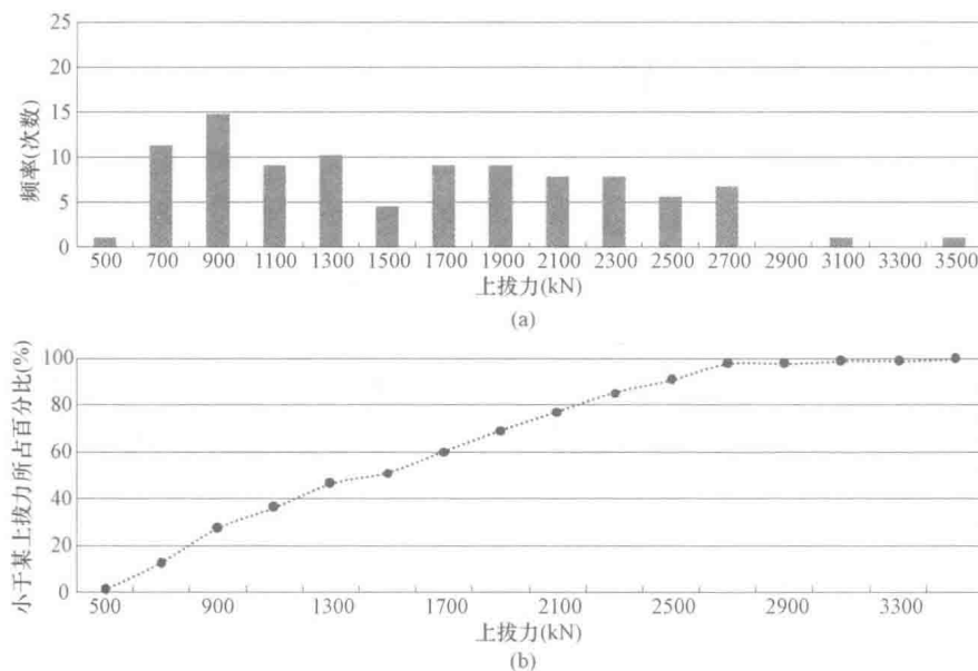
图 4.2-6 750kV 电压等级直线塔基础上拔力分布直方图及累积分布曲线 (a) 基础上拔力分布直方图；(b) 基础上拔力累积分布曲线
