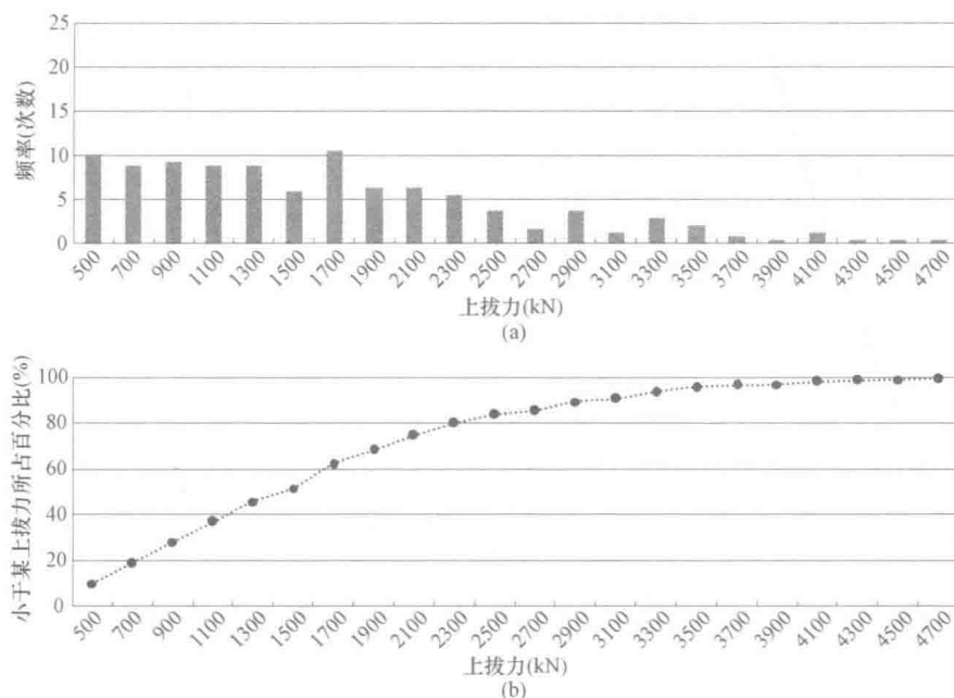
图 4.2-5 500kV 电压等级直线塔基础上拔力分布直方图及累积分布曲线 (a) 基础上拔力分布直方图；(b) 基础上拔力累积分布曲线
