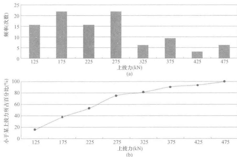
图 4.2-1 66kV 电压等级直线塔基础上拔力分布直方图及累积分布曲线 (a) 基础上拔力分布直方图; (b) 基础上拔力累积分布曲线
