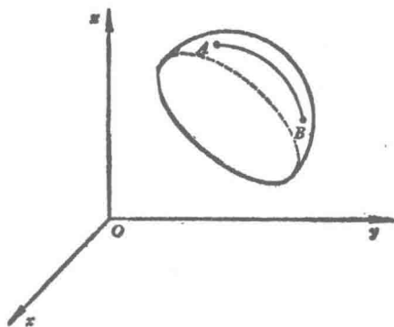
图 1.2 曲面上两点 A, B 间的短程线
