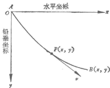
图 1.1 最速降线, A, B 两点固定, A 点和坐标原点重合
